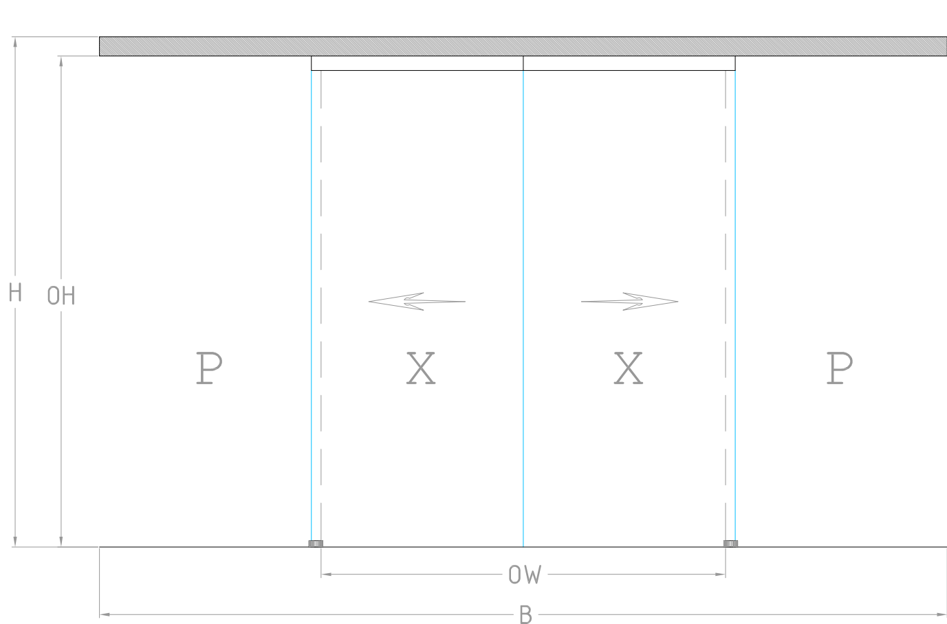
Alzado
