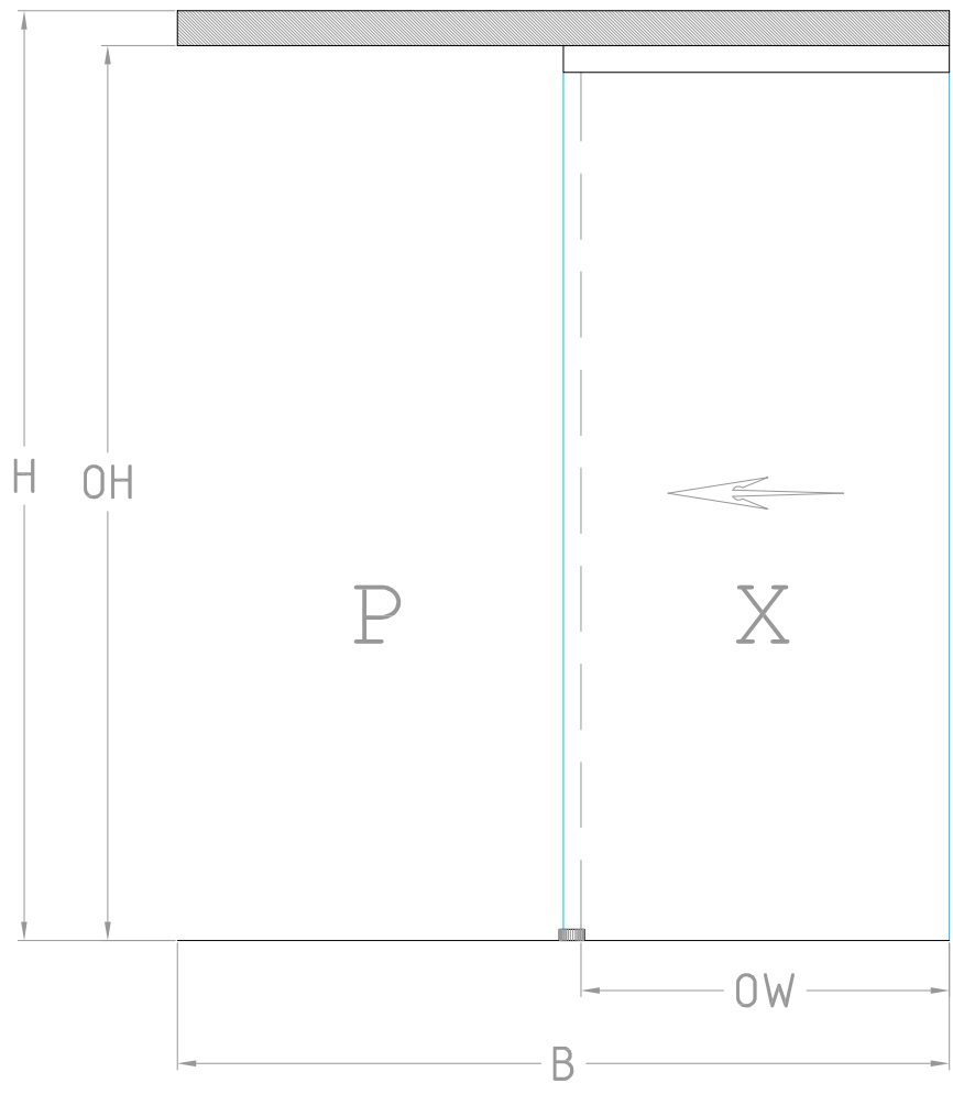
Alzado
