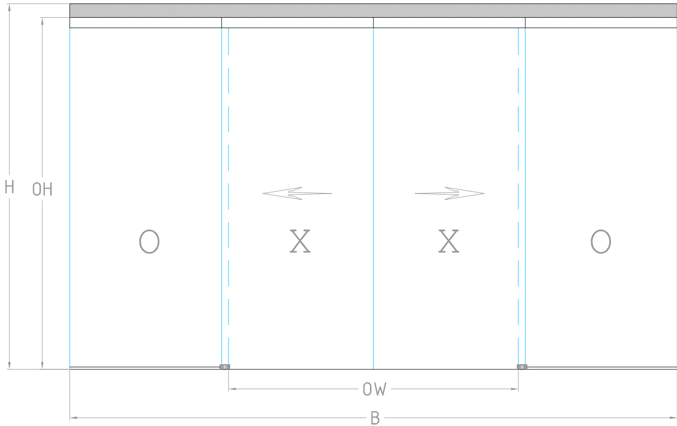
Alzado
