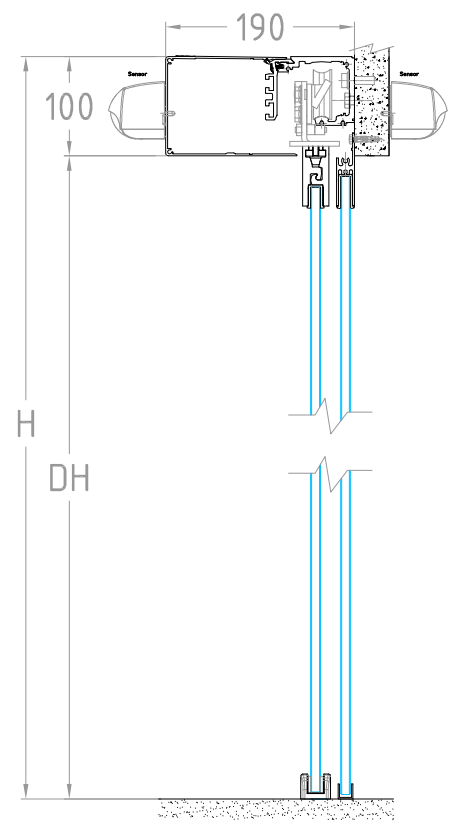
Corte
