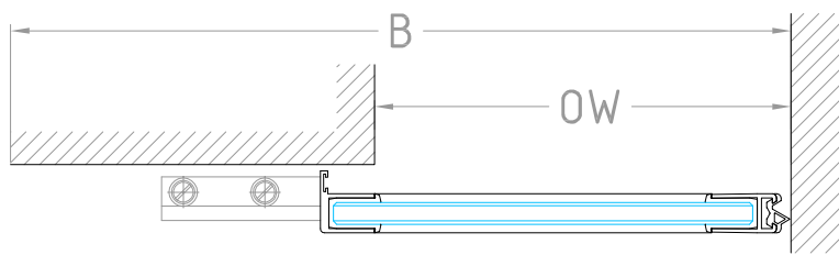
Alzado
