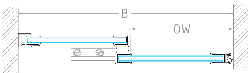
Planta
