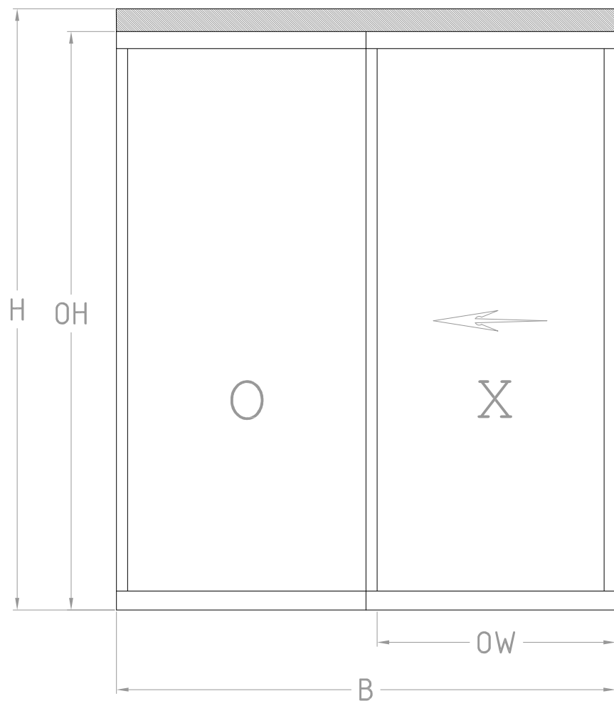
Alzado
