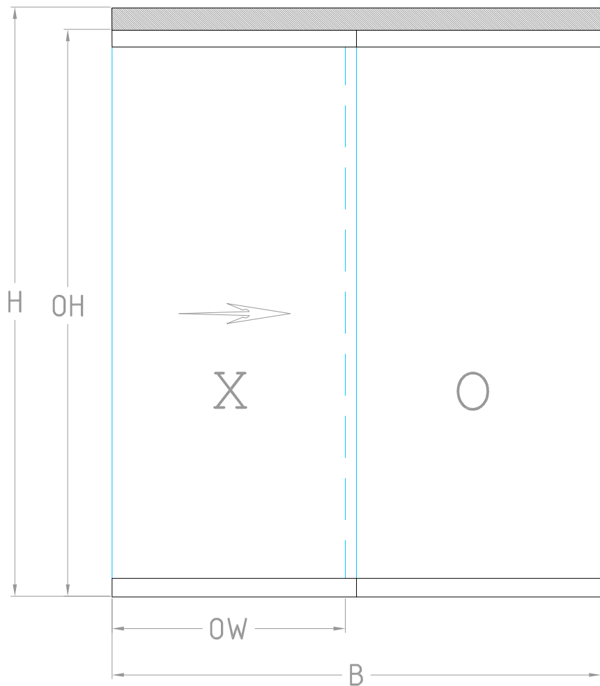
Alzado
